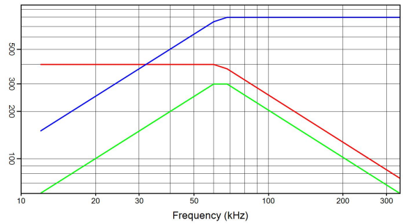
CSP 305A 5 μF 400 V rms 800 A rms 300 kVA r I(A) — Q(kVA r ) — V rms
