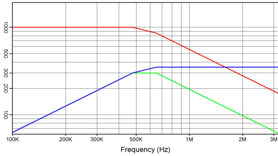
CSP 305A 0.1 μF 1000 V rms 350 A rms 300 kVA r I(A) — Q(kVA r ) — V rms
