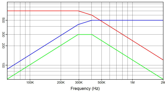
CSP 305A 0.33 μF 700 V rms 500 A rms 300 kVA r I(A) — Q(kVA r ) — V rms
