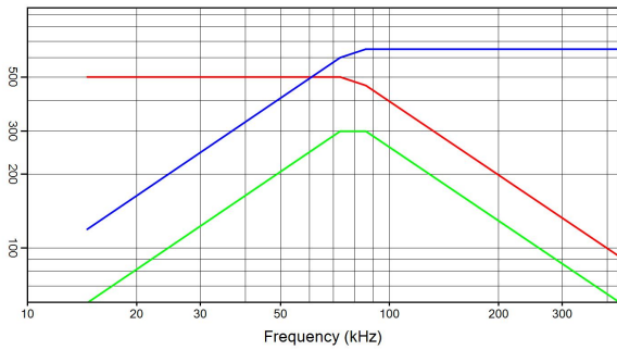
CSP 305A 2.6 μF 500 V rms 650 A rms 300 kVA r I(A) — Q(kVA r ) — V rms
